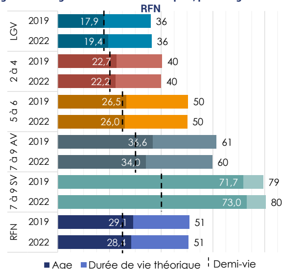
Figure 1.2 – Âge et durée de vie théoriques, par catégorie de voie du RFN
